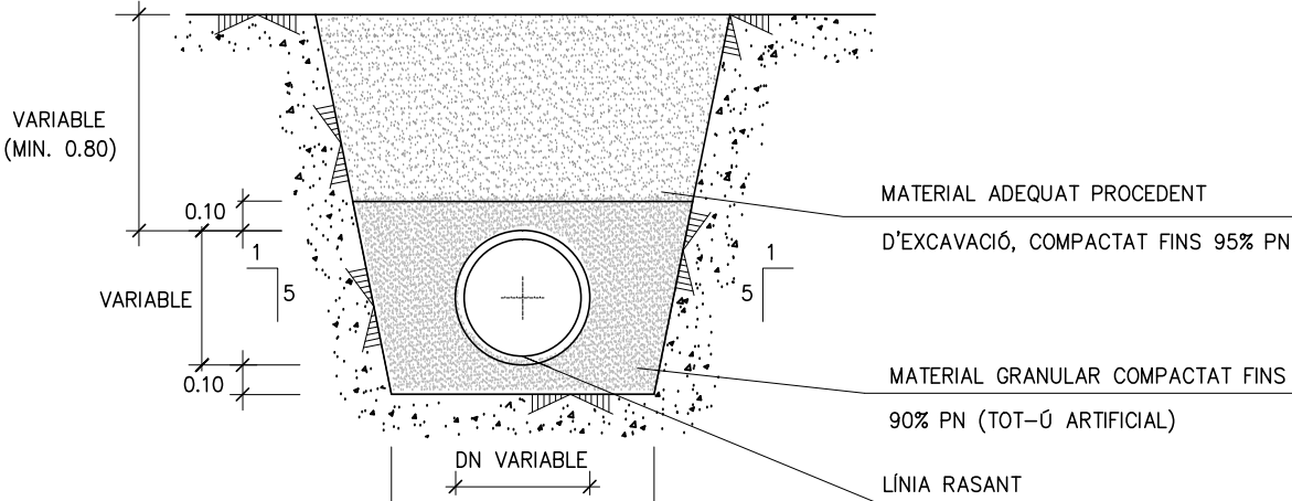
RASA TIPUS. XARXA ABASTAMENT D'AIGUA
