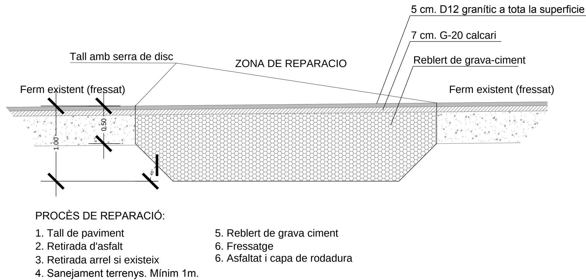
DETALL REPARACIO DEL PAVIMENT DE CALÇADA EXISTENT
