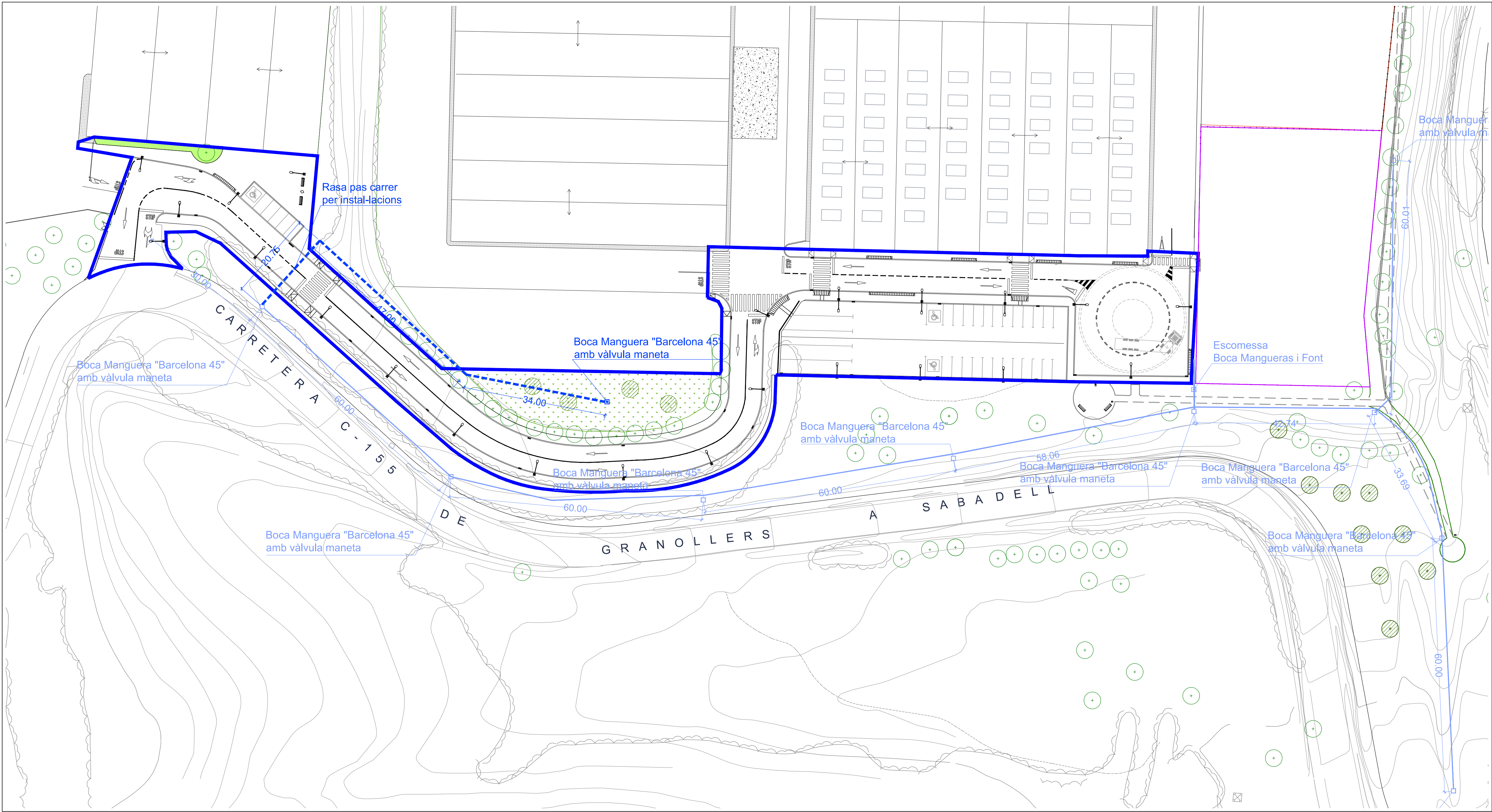
XARXA DE REC AUTOMÀTIC E:1/500
