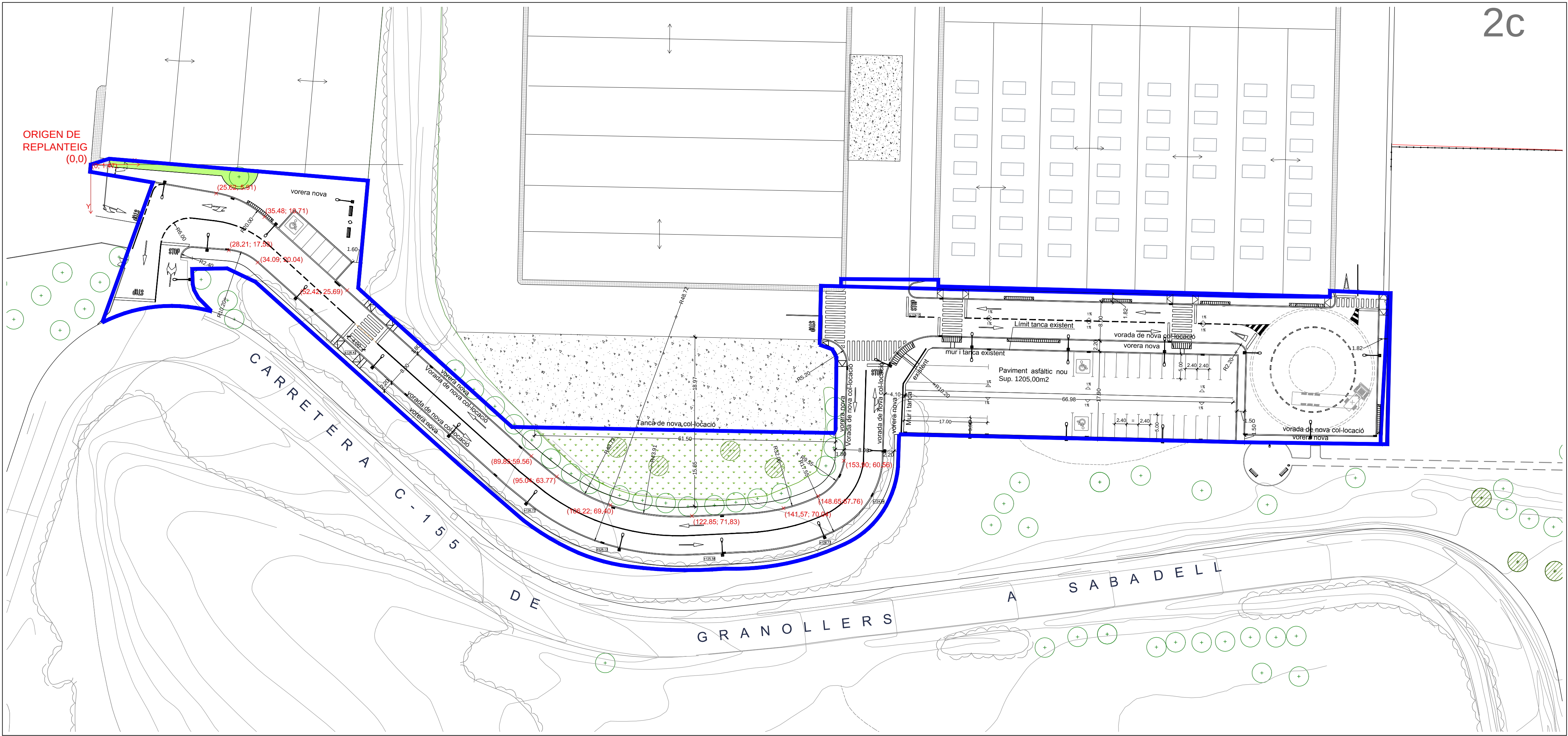
DEFINICIÓ GEOMÈTRICA E:1/500
